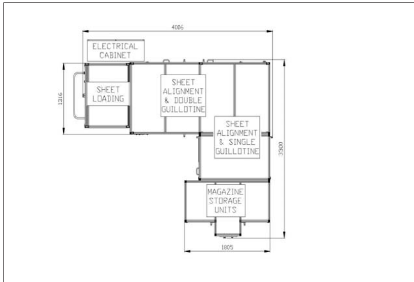
ODG502 DOUBLE GUILLOTINE FOOTPRINT
