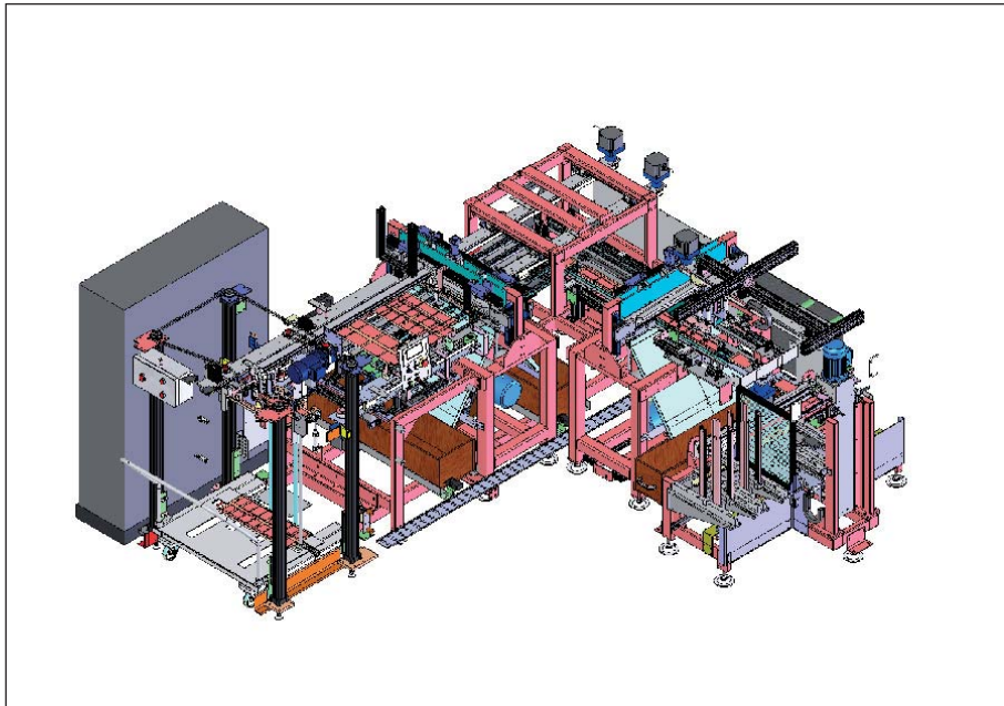
ODG502 DOUBLE GUILLOTINE FOOTPRINT
