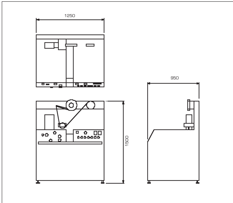
OHR 100 FOOTPRINT
